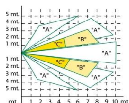
VISTA IN PIANTA
